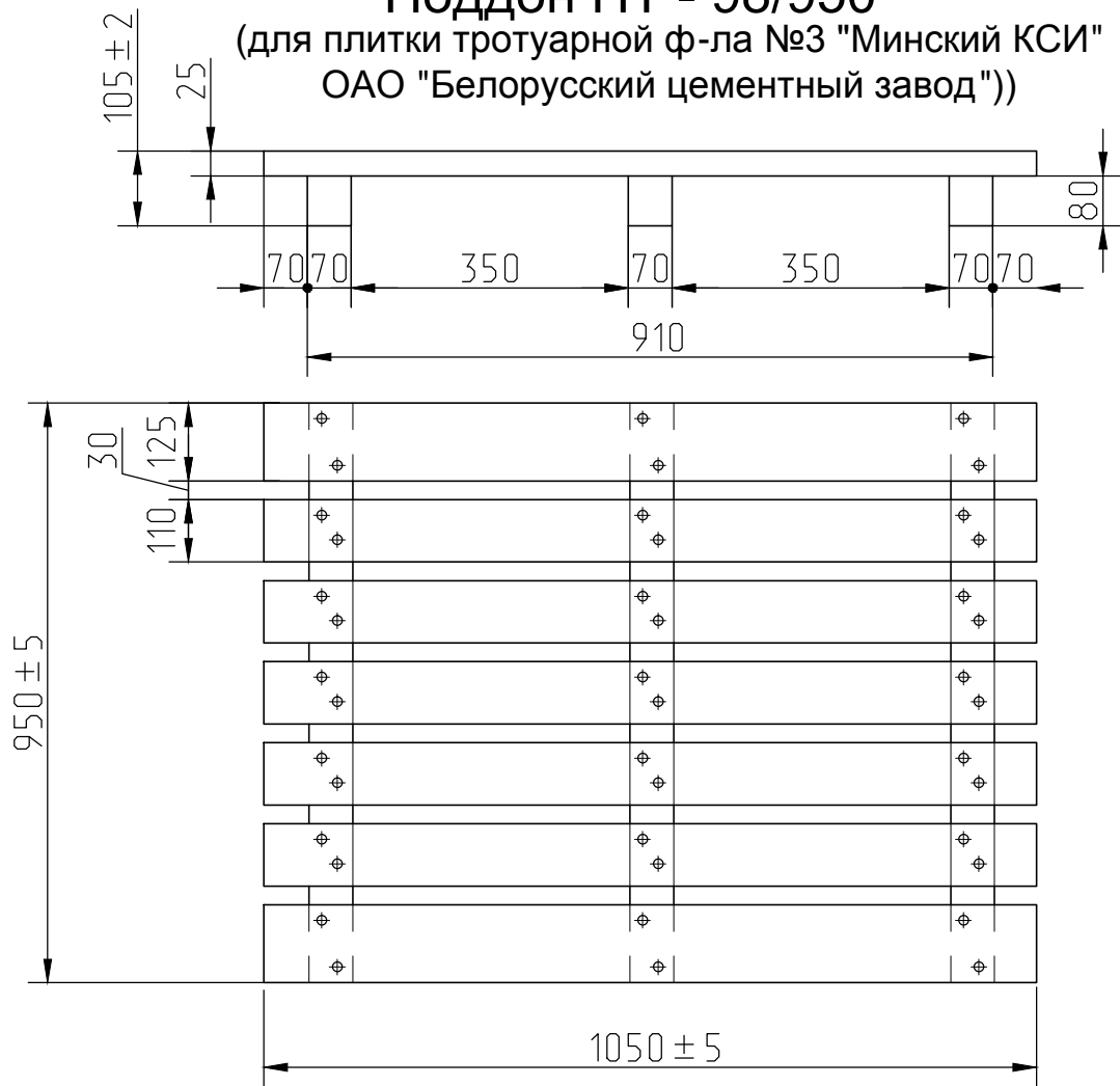
Размеры поддона
